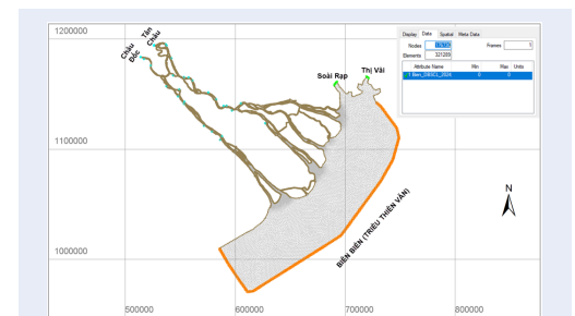
Hình 3: Miền lưới tính toán và vị trí các biên trong TELEMAC2D
