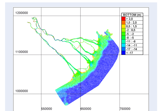
Hình 4: Địa hình lòng dẫn khu vực nghiên cứu
